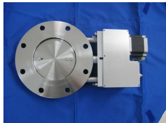
ISO100フランジ スロットルバルブ 外観
